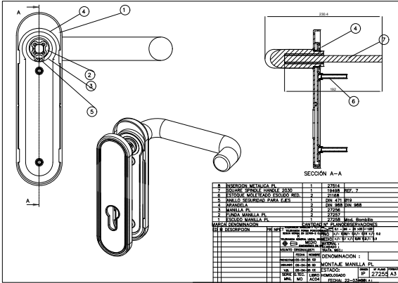
DETALLE DE MANIJA
