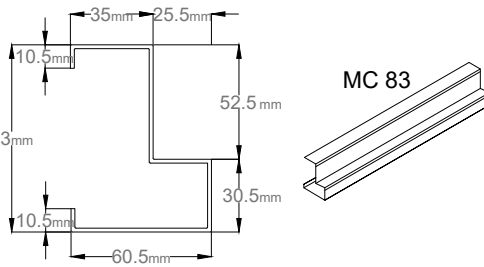
DETALLE DEL PERFIL DEL MARCO
