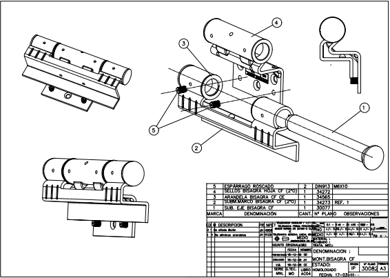
DETALLE DE BISAGRA
