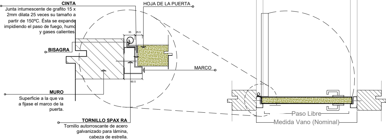
PROYECCION DE ABATIMIENTO
