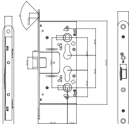
DETALLE DE CERRADURA CF60
